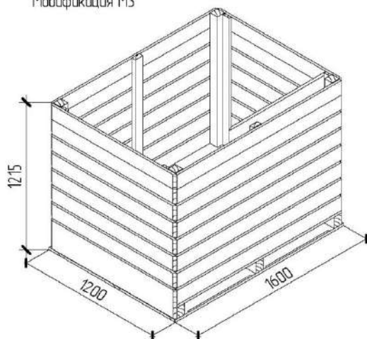
Модификация М3
